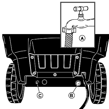
Collegamento idrico.
