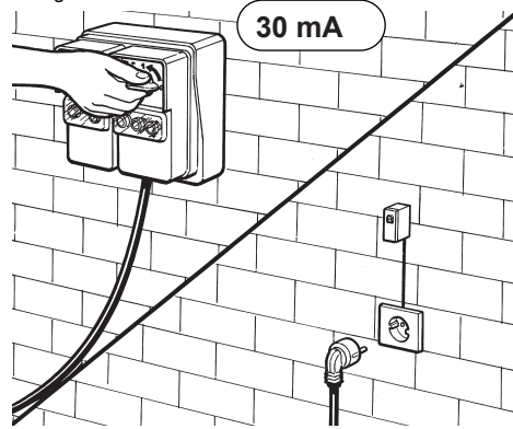
Collegamento elettrico.
