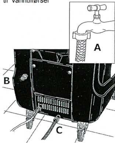
Tilkobling til vanntilførsel
