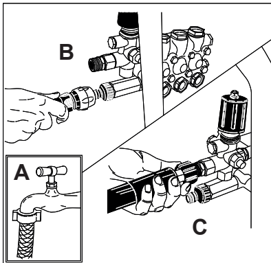
Vesikytkentä.
