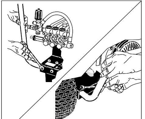
Kahvojen asennus.
