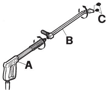
Kärkiosan asentaminen.
